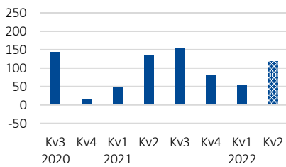
KASSAFLÖDE FRÅN DEN LÖPANDE VERKSAMHETEN, MSEK
